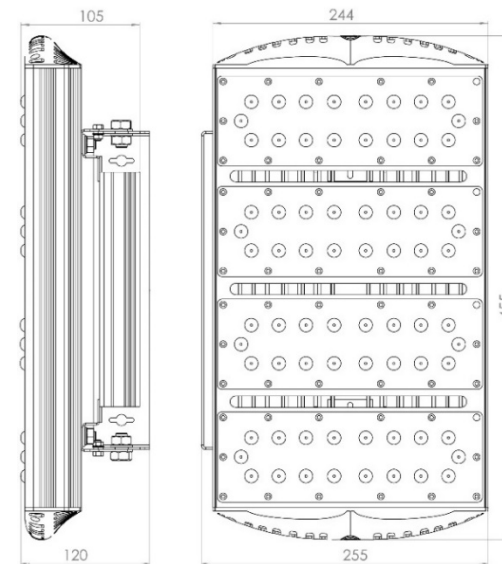
ГАБАРИТНЫЙ ЧЕРТЕЖ
