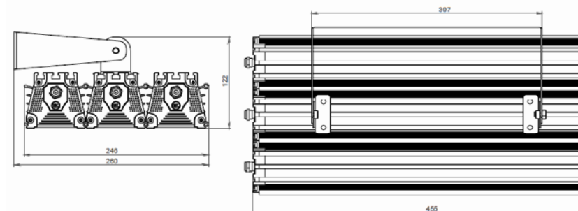
ГАБАРИТНЫЙ ЧЕРТЕЖ
