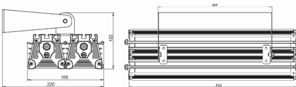
ГАБАРИТНЫЙ ЧЕРТЕЖ
