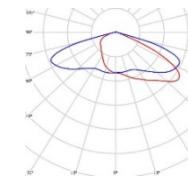
КСС Ш
