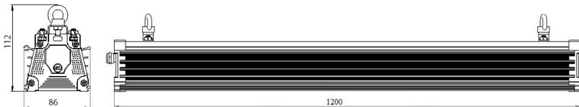
ГАБАРИТНЫЙ ЧЕРТЕЖ
